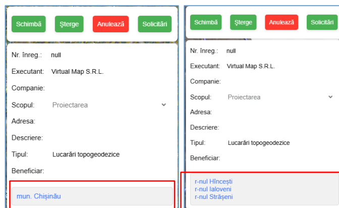
Figura 5: Formular completat.
