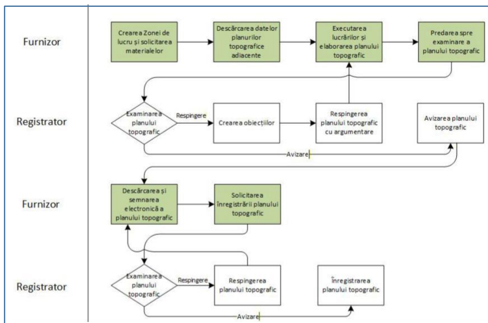
Schema 1: Procesul tehnologic executat pentru a înregistra lucrarea topogeodezică
